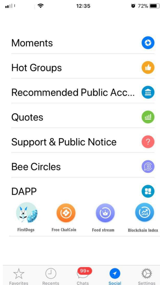
Image2: BeeChat UI
